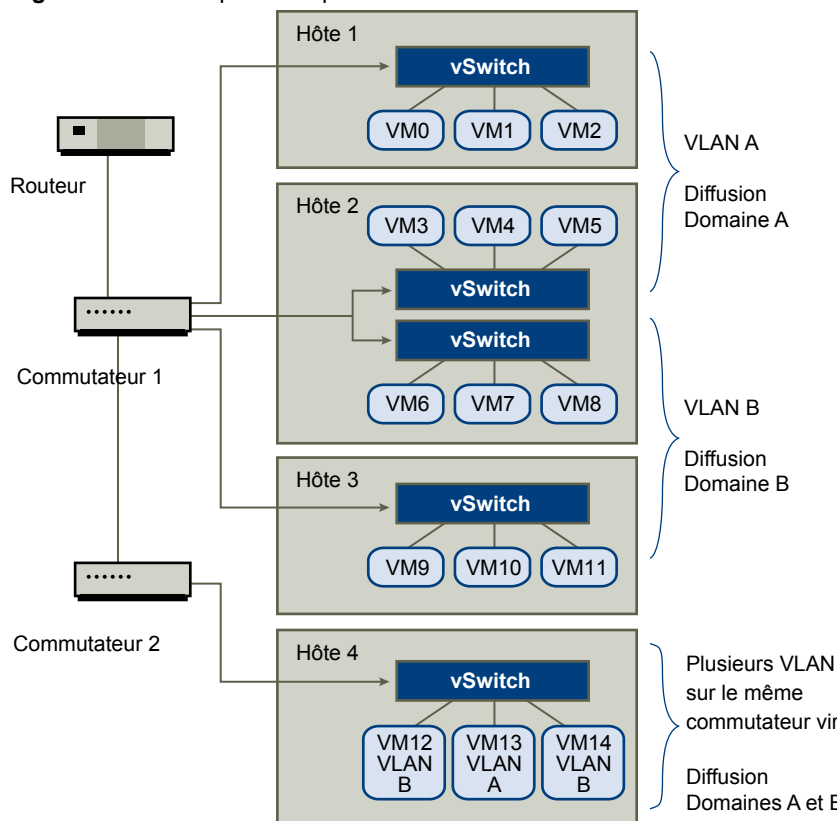
Figure 12-4. Exemple de disposition de VLAN
